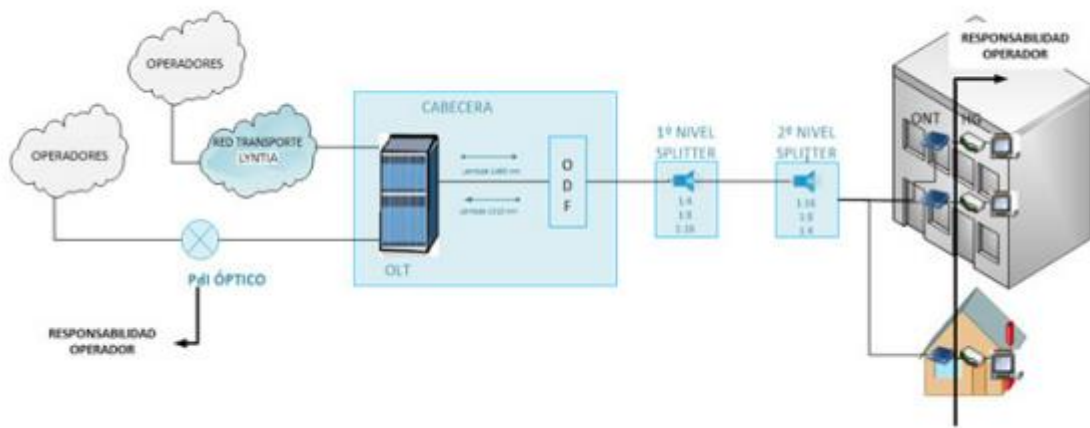
Figura 2 Arquitectura general de la red, opción 2
